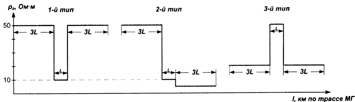
Рисунок 1 - Типы чередования грунтов с различными удельными сопротивлениями
