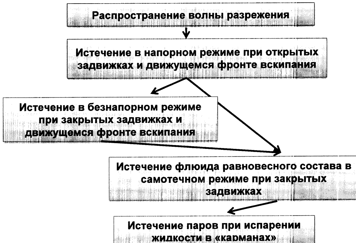
Рисунок 2 – Стадии истечения нестабильной жидкости при гильотинном разрыве КП/ПП
