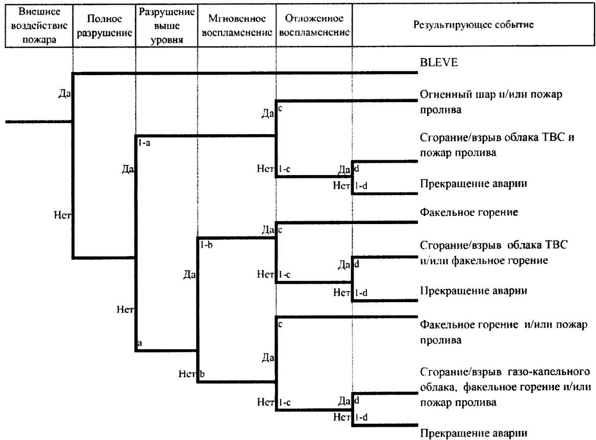
Рис. 2. Дерево событий при разгерметизации емкостного оборудования с ШФЛУ
