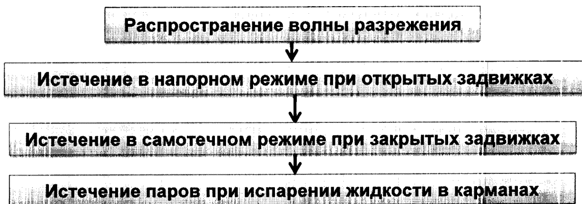
Рисунок 1 – Стадии истечения стабильной жидкости при гильотинном разрыве
